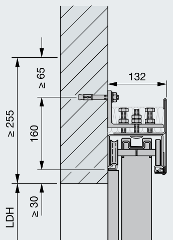
Απευθείας συναρμολόγηση οροφής με τεχνητό πρέκι
