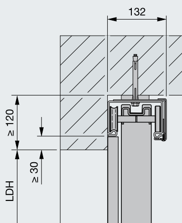
Αναρτώμενη συναρμολόγηση στην οροφή (μόνο στην περιοχή ρύθμισης)
