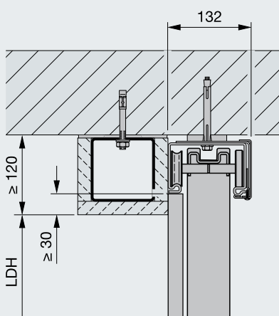
Απευθείας συναρμολόγηση οροφής με τεχνητό πρέκι
