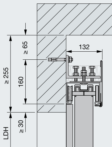
Απευθείας συναρμολόγηση οροφής
