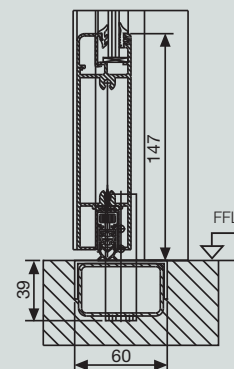
Στάνταρ χωρίς κατοκάσι, κατόπιν ζητήσεως με αυτόματο ανεμοφράκτη
