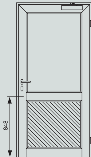
Κατόπιν ζητήσεως, με οριζόντιο προφίλ και μηχανισμούς επαναφοράς (για τις καπνοστεγής πόρτες, ο μηχανισμός επαναφοράς είναι
