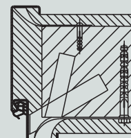
Προφίλ πλαισίου που τοποθετείτε σε τοιχοδομία ενυόμενα ελαστικά / στηρίγματα αγκύρωσης
